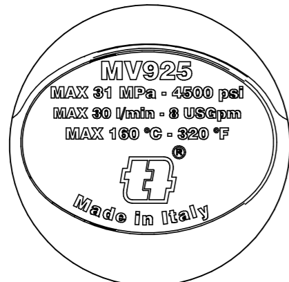
DETTAGLIO-DETAIL A
